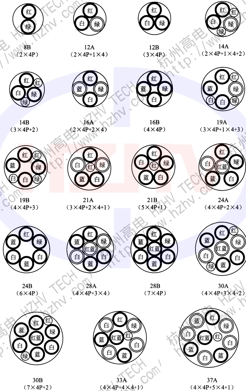
图 B.1 电缆 A 端排列示意图
