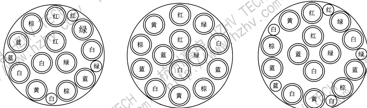
52芯 (12×4+4)
