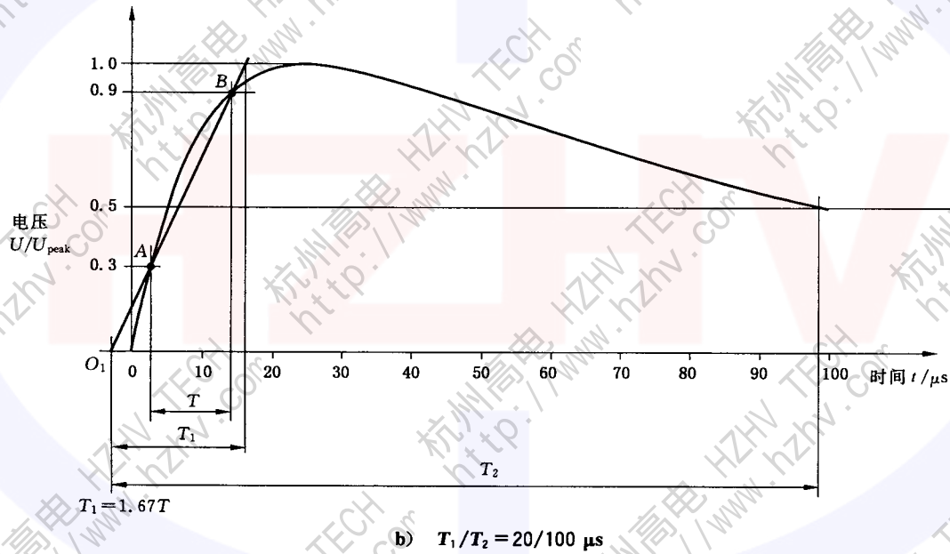
图 1 非振荡型雷电冲击波形
