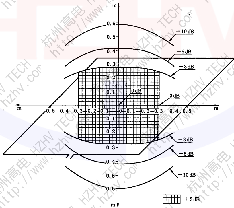
图 B.3 正方形感应线圈(边长为 1 m)在中央垂直平面上产生的磁场的 3 dB 区域(垂直于线圈平面的分量)
