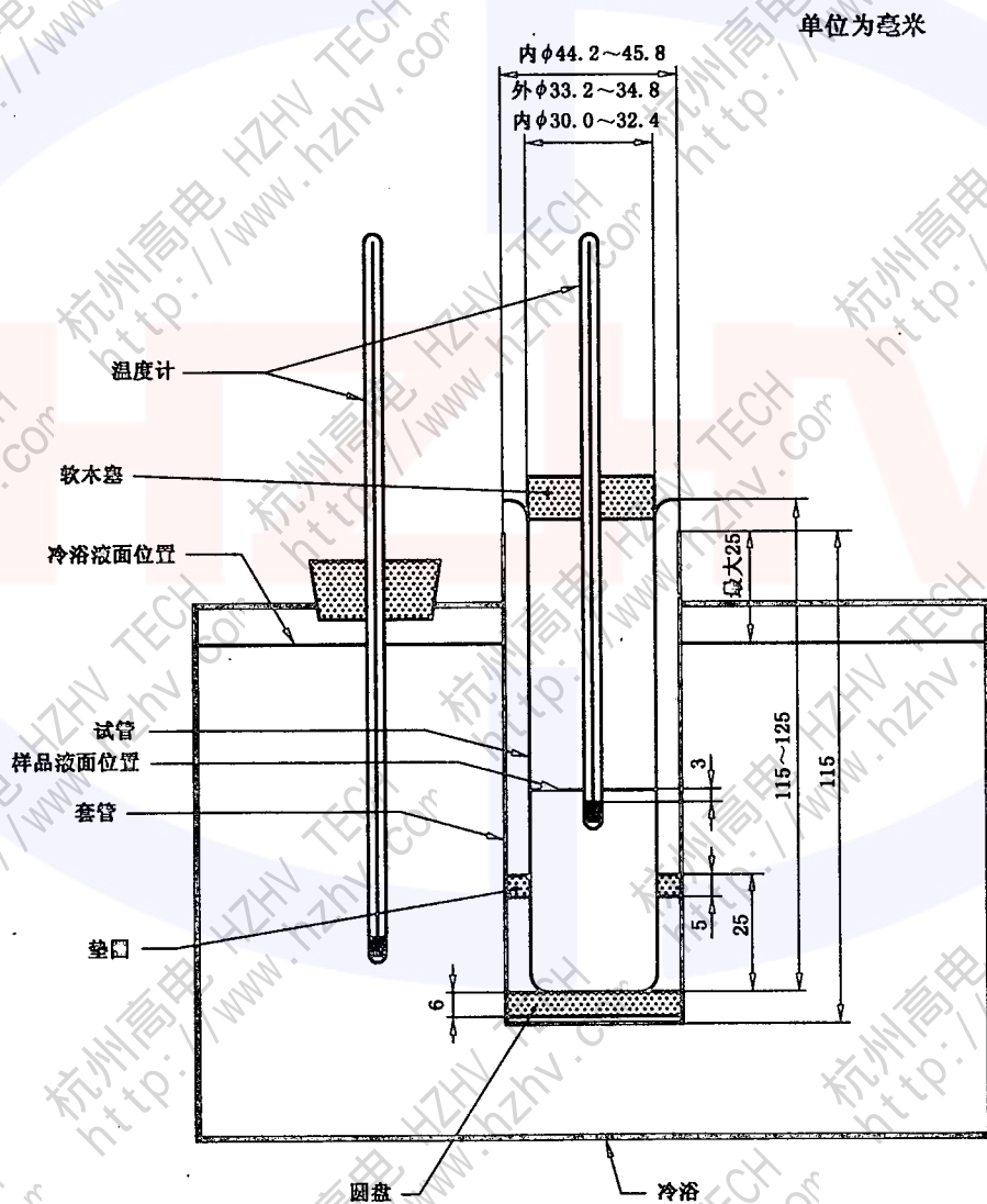
图1 倾点测定仪
